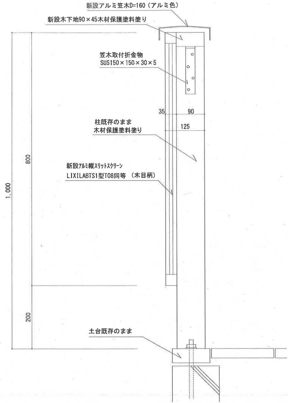
新設手摺り断面図 S:1/5
