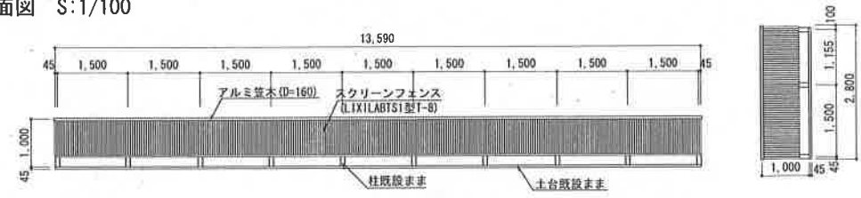
新設スクリーン手摺 姿図 S:1/100
