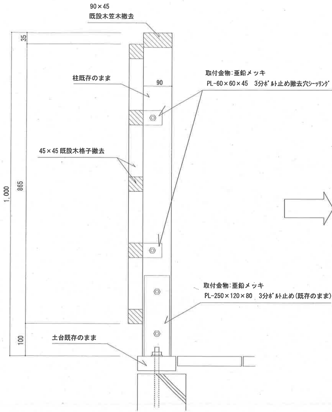
既設手摺り断面図 S:1/5
